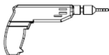
Perceuse-visseuse
